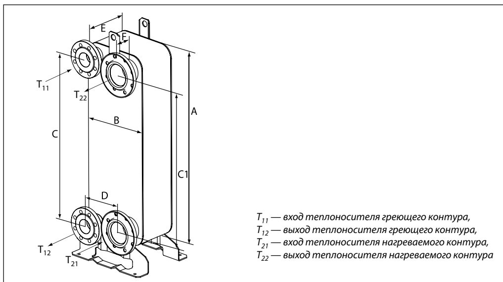
Паяный теплообменник XB 70L
